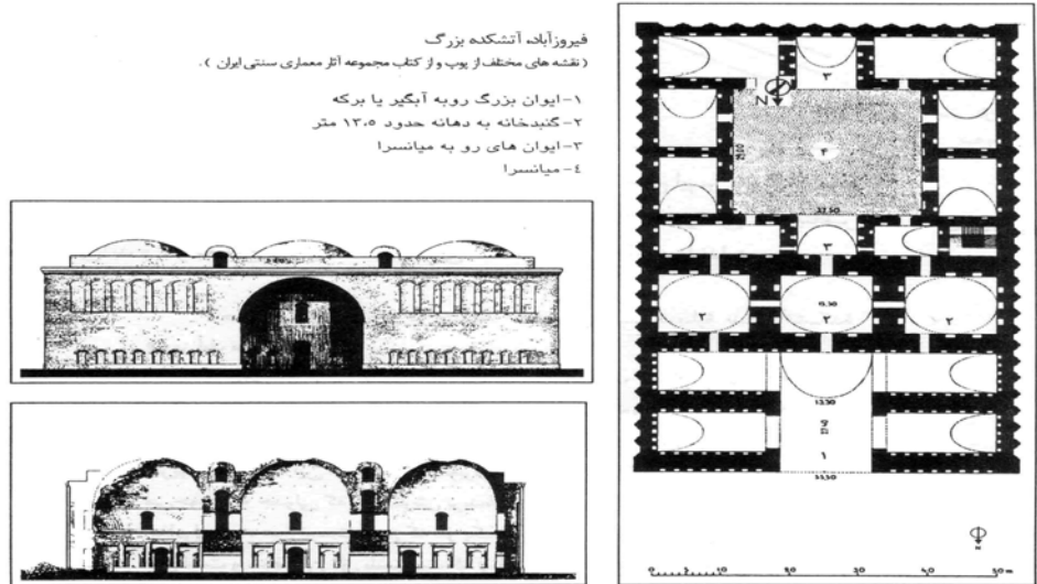
آتشکده فیروزآباد، نمای اصلی آتشکده فیروزآباد، برش از سه کنیخانه.
