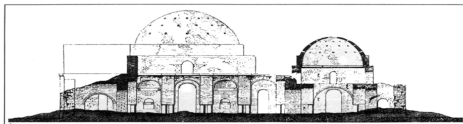
کاخ سروستان، برش از اتاق کعبه دار کوچک (از مجموعه اثر معماری سنی ایران).
